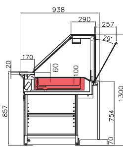
VKBBM - VD banho-maria bain marie bain-marie baño maria
