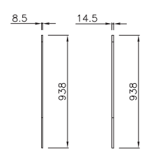
8,5/14,5mm lat. de acoplamento coupling panel jouis d'assemblage lat. de acoplamiento
