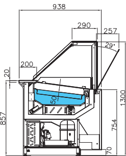
VKBSF - VD semifrio frozen desert entremets glacés semi frio
