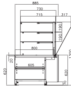
TVKB - VD torre de vidro tower glass tour vitrée torre de vidrio
