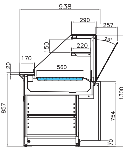
VKBTRS - VD 3M2 tampo refrigerado refrigerated deck exposition réfrigéré tablero refrigerado
