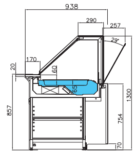
VKBSLS - VD 3M2 saladas superior upper vent. salads salades supérieure ensaladas superior
