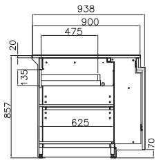
CXKB1N caixa de saída support case meuble caisse caja de salida
